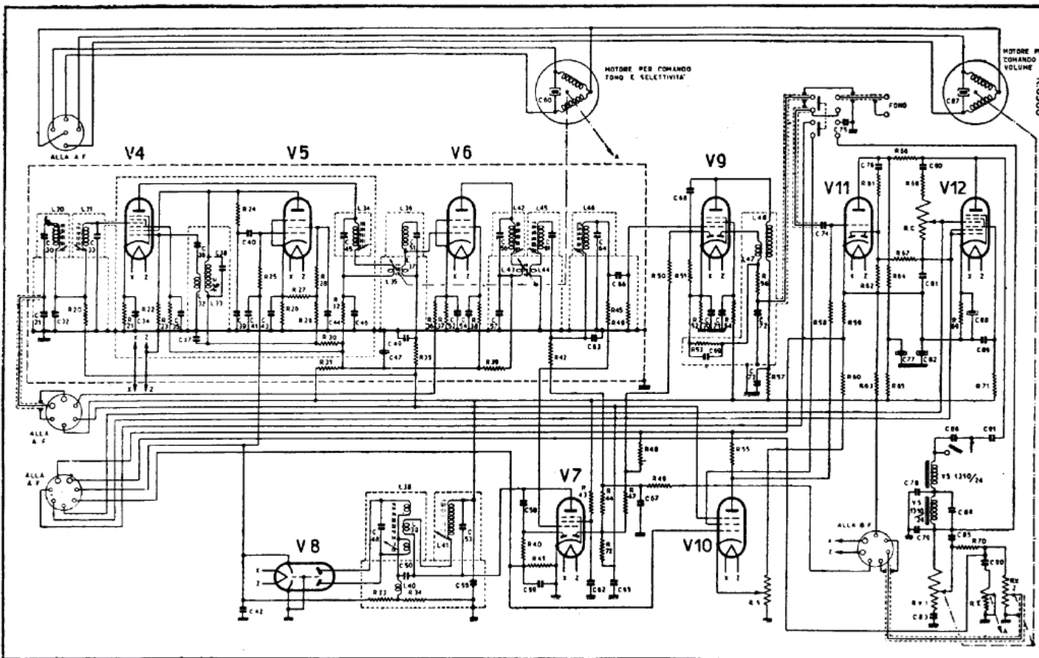
171. — PHONOLA (S. A. FIMI). — Mod. 1800. — Compl. MF. — Produzione 1939. — Media frequenza: 470 kHz.
